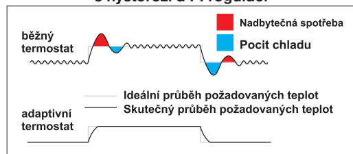
Rozdíl mezi nastavením termostatu s hysterezi a PI regulací
